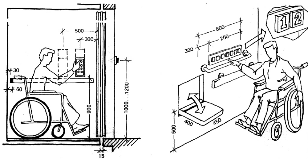
Lifta/ pacēlāja vadības pults izvietojums.
